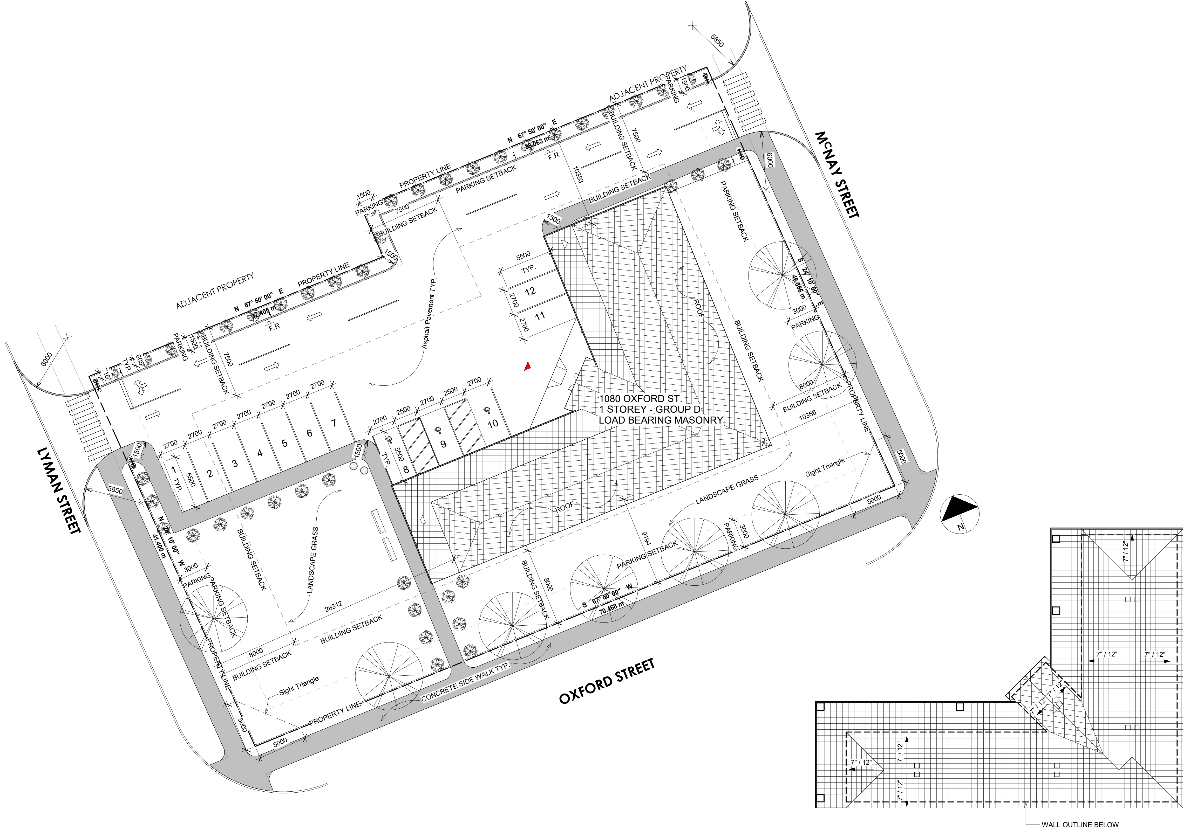
1 SITE PLAN 1 : 200
