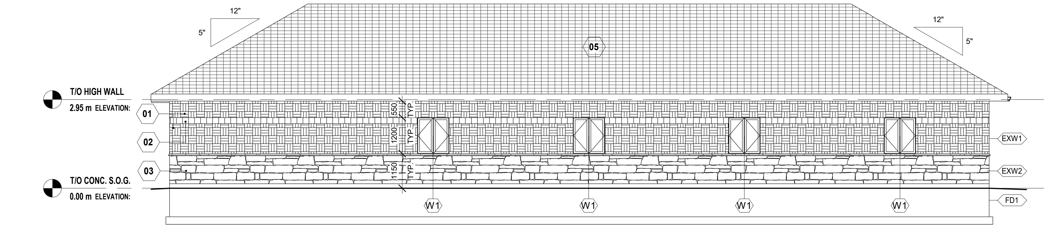
3 EAST 1 : 75
